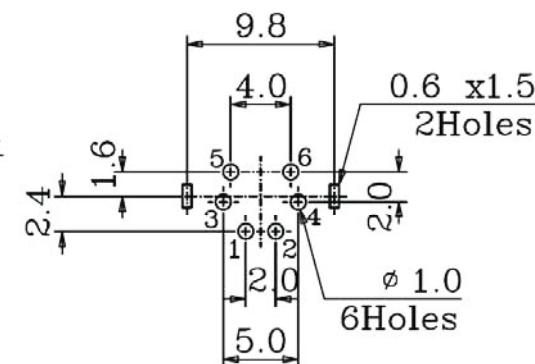
P.C.B. HOLE LAYOUT
