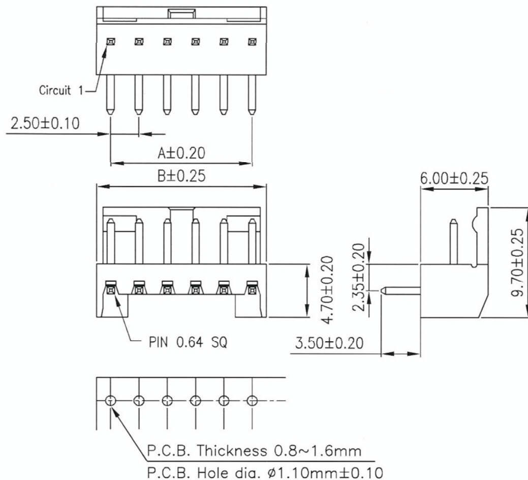
P.C.B. LAYOUT
