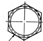
1/2-28 UNEF-28 CLAMP NUT
