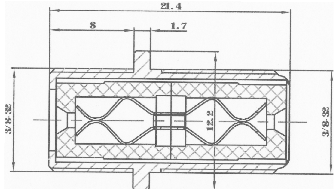
F-Adapter, Kupplung auf Kupplung
