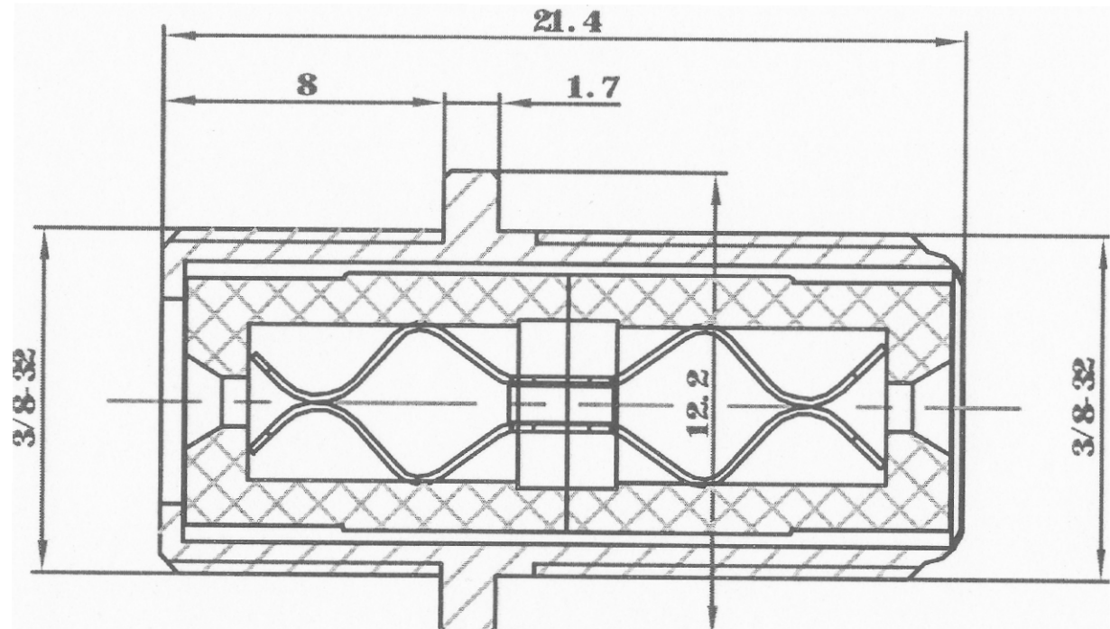
F-Adapter, Kupplung auf Kupplung
