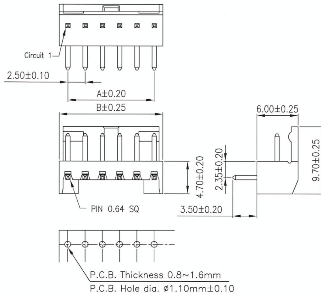
P.C.B. LAYOUT
