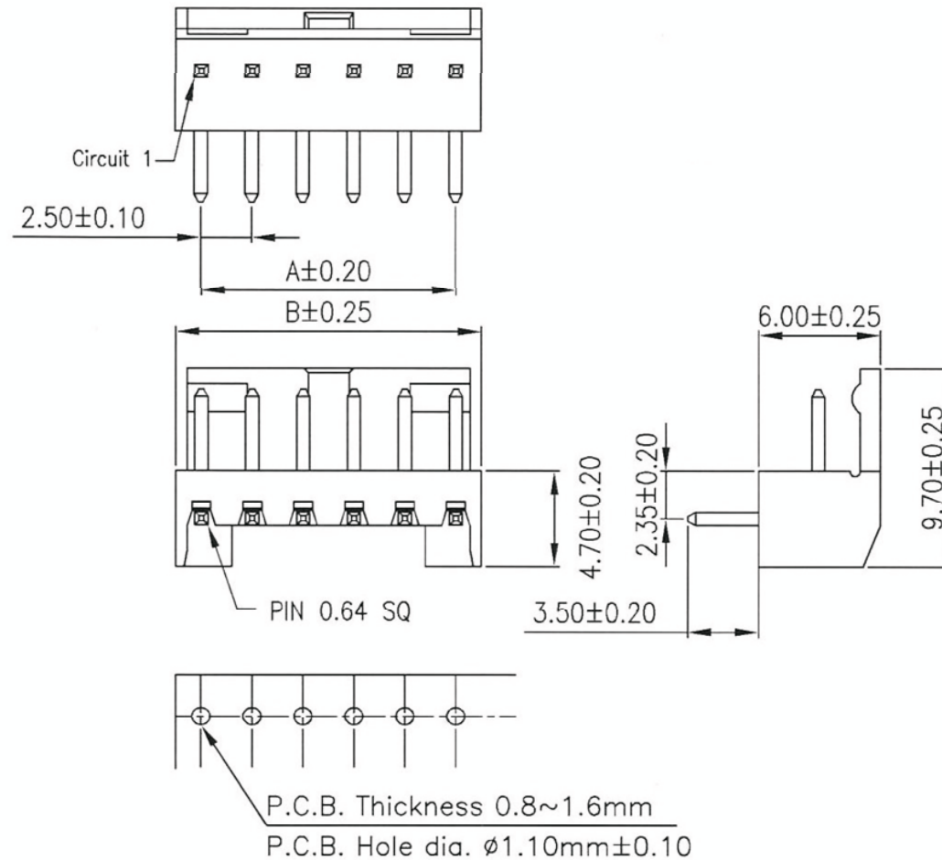
P.C.B. LAYOUT
