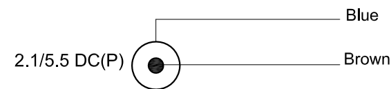
Wiring
