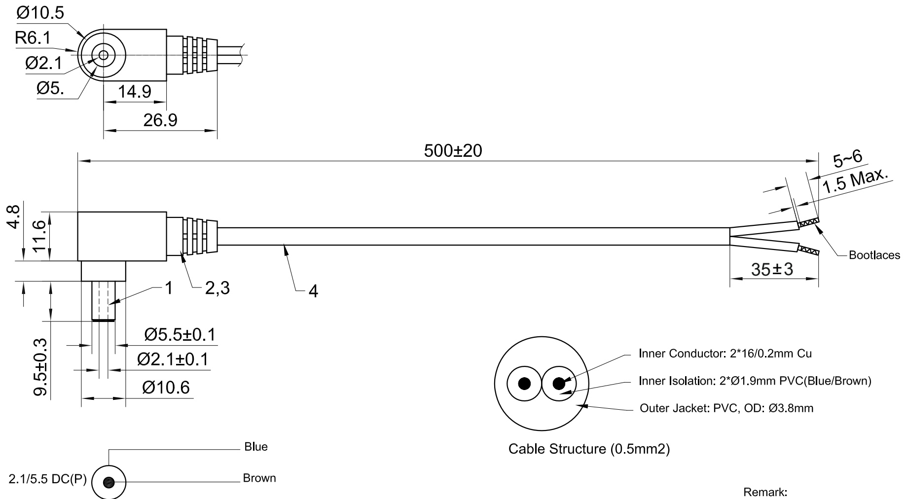
Wiring
